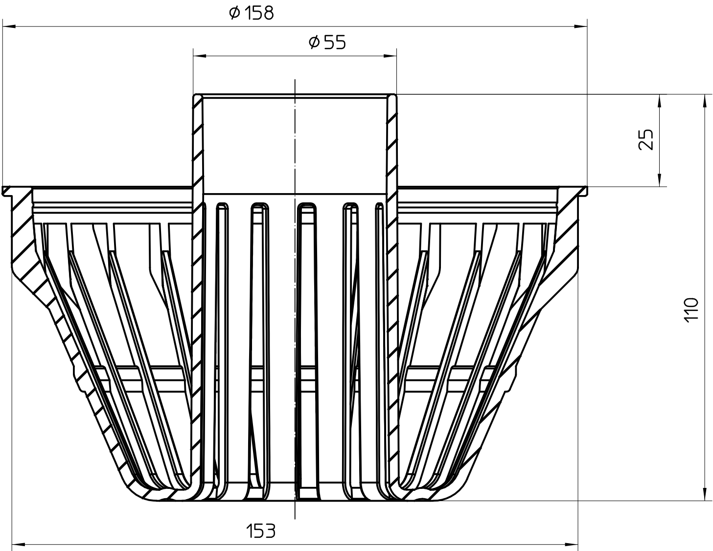
Schnitt A-A
