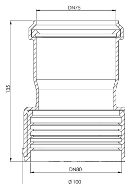
Techn. Zg. HL9/7/8
