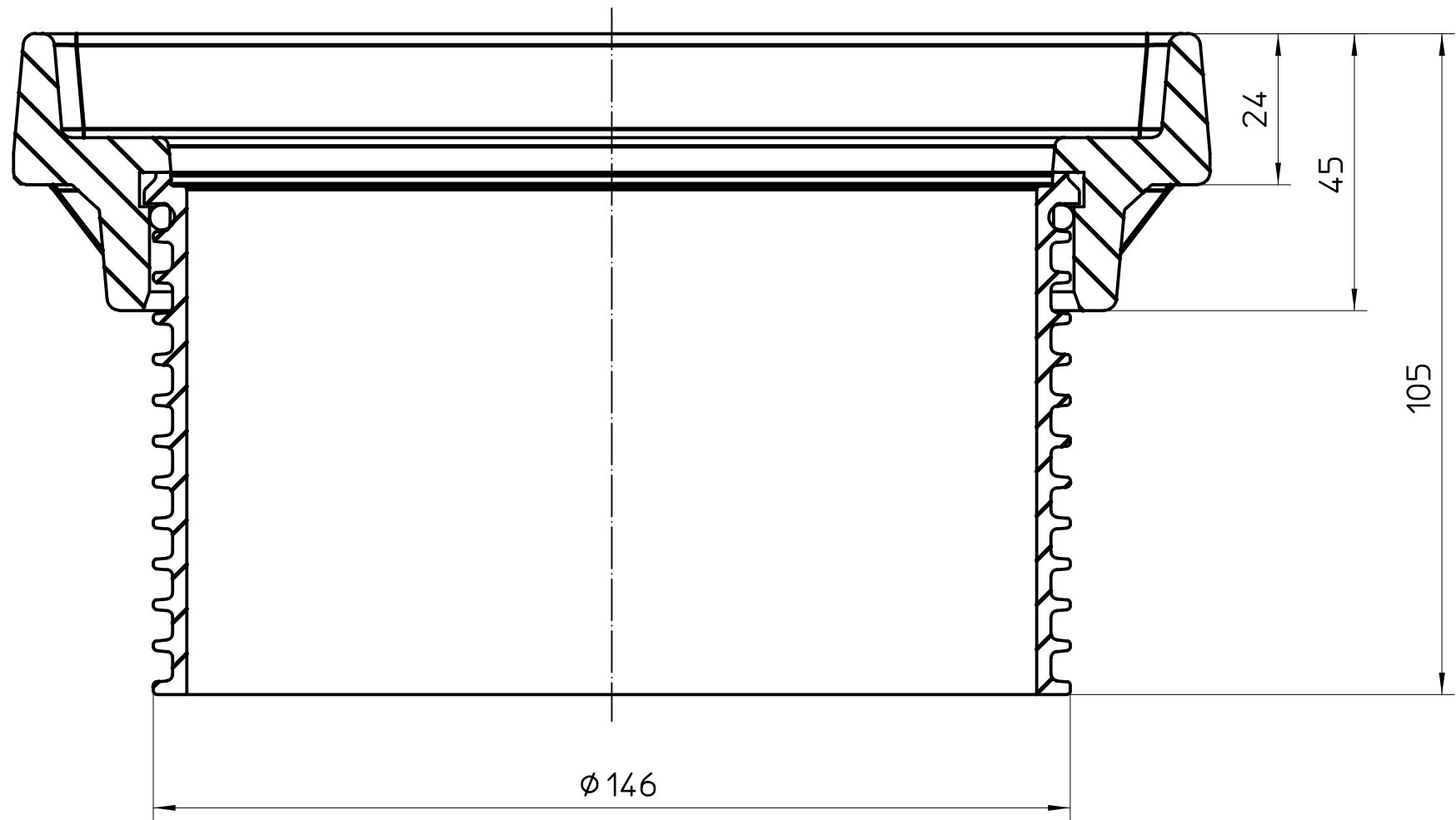
Schnitt A-A
