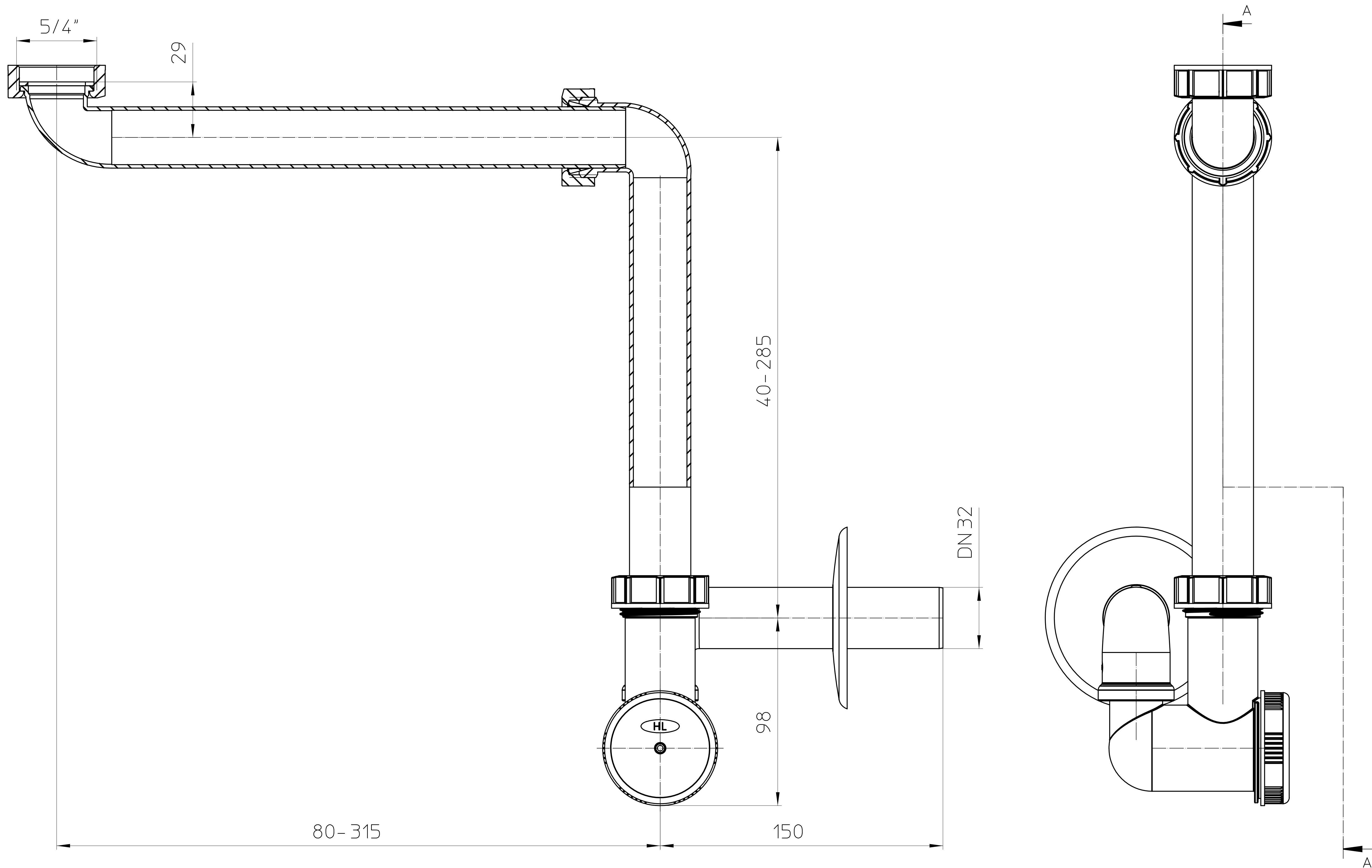
Schnitt A-A
