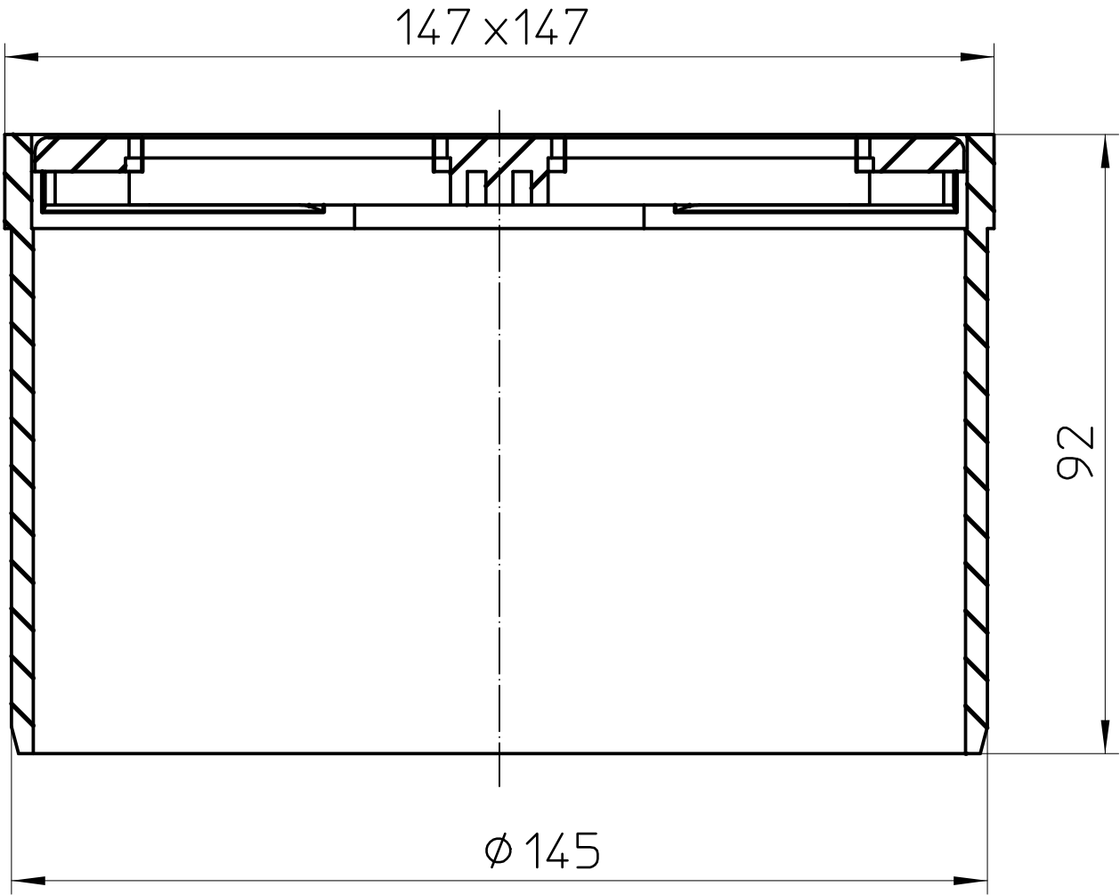
Schnitt A-A
